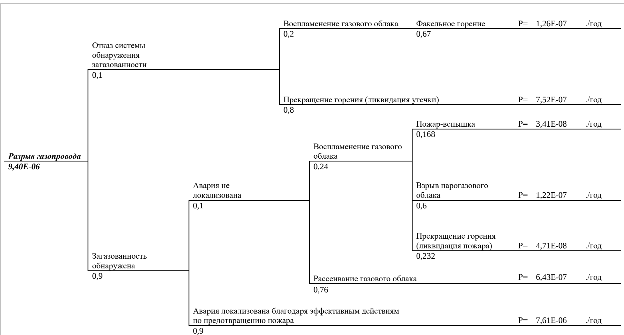
Рисунок 3.3.8 – «Дерево событий» при реализации сценария С42.
