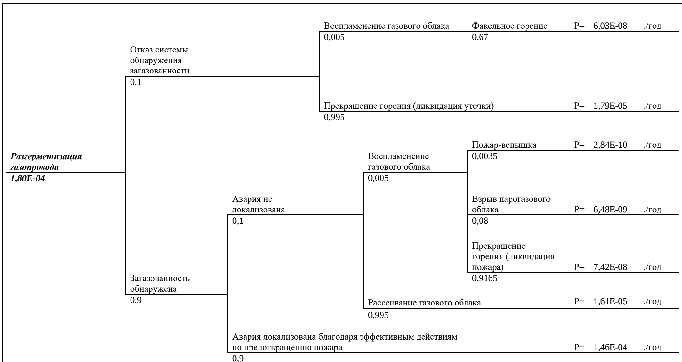
Рисунок 3.3.5 – «Дерево событий» при реализации сценария С31.
