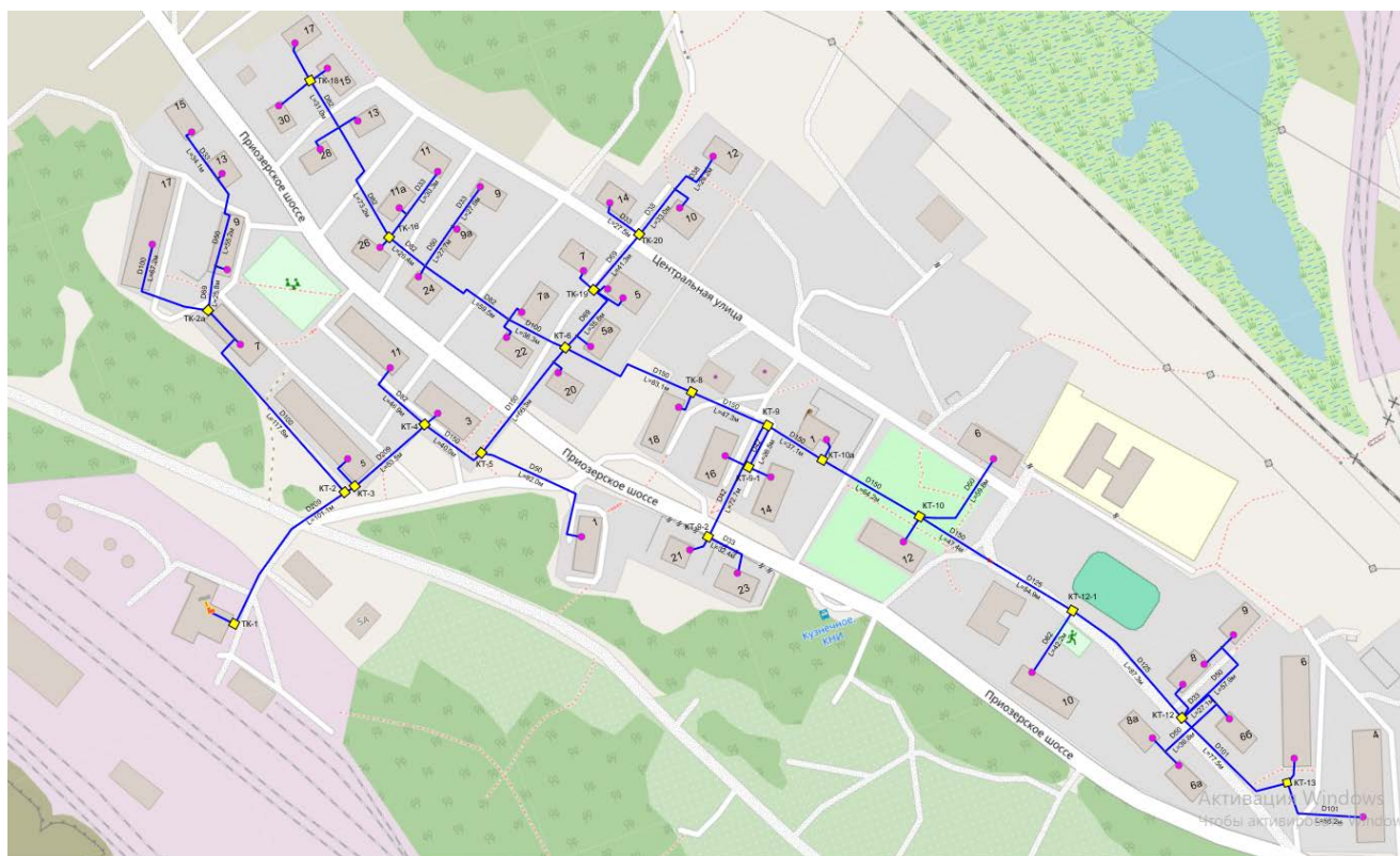
Рисунок 10.4.2 – Зона действия Котельная №2 «КИН» в нормальном режиме теплоснабжения
