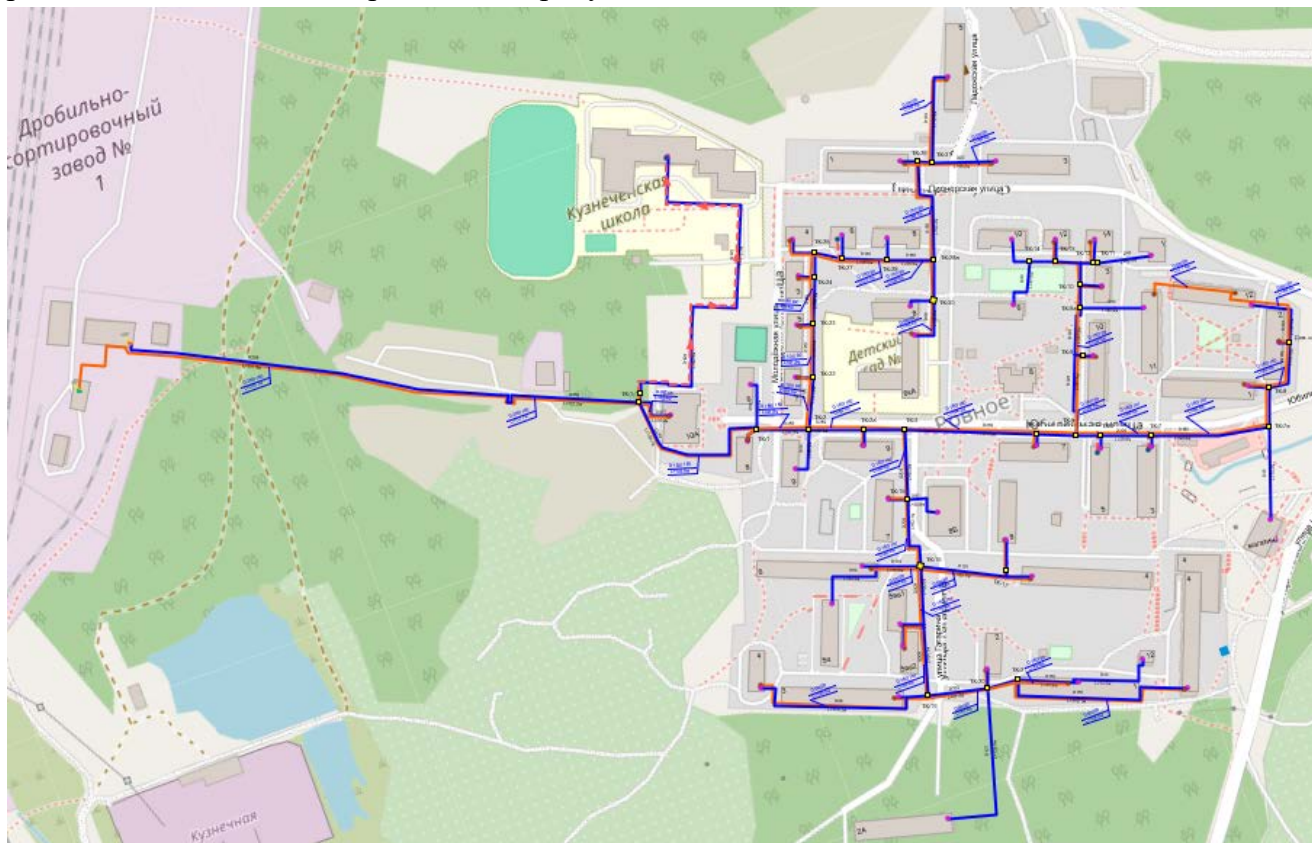
Рисунок 10.4.1 – Зона действия Котельная №1 «Ровное» в нормальном режиме теплоснабжения
